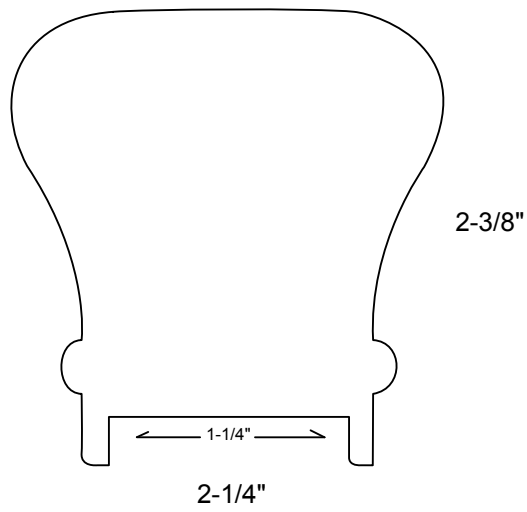
6010P Handrail
