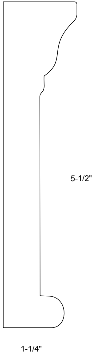
HDRCSG Architrave
